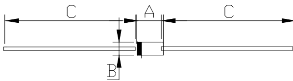
DO-204AL(DO-41)
