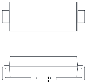
DO-214AC(SMA)
